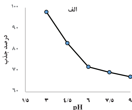
شکل ۳- تأثیر pH (الف) و زمان تماس (ب) بر فرایند جذب آرسنات توسط جاذب nZVI-Chitosan برای غلظت اولیه 2 mg/L آرسنات و دز جاذب 2 g/L
