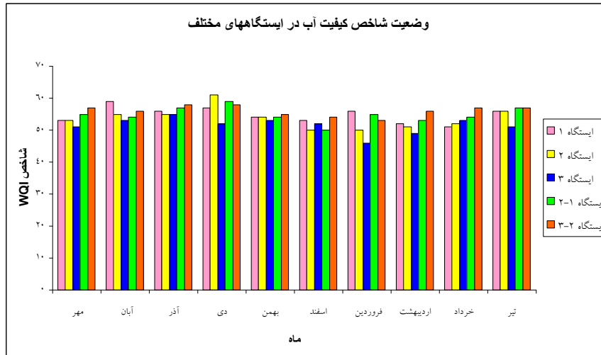
شکل ۲- وضعیت شاخص کیفیت آب (WQI) در ماه‌های مختلف سال و در ایستگاه‌های مختلف
