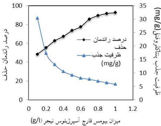
شکل ۶. اثر مقدار بیومس بر فرایند جذب (pH = ۵، زمان تماس h، غلظت ۲۵ mg/L و سرعت اختلاط ۱۲۰ rpm)
