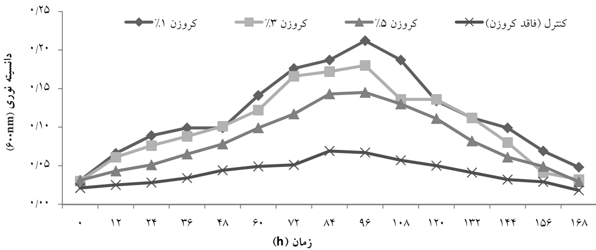
نمودار ۳- دانسیته نوری سراسیا مارسسنس در غلظت‌های مختلف کروزن
