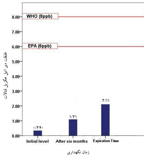
شکل ۲- تفاوت میان بیشینه غلظت دی اتیل هگزیل فتالات (برحسب میکروگرم بر لیتر) در روز اول تولید آب‌های بطری شده با میان و پایان دوره مصرف و مقایسه آن با حد مجاز اعلام شده توسط EPA و WHO ( 6 \mu\text{g/L} و 8 \mu\text{g/L} ).
