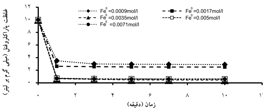
شکل ۳: تاثیر Fe^0 بر کارایی حذف پاراکلروفنل توسط فرایند شبه فتوتون ( H_2O_2=0/0.002mol/L , pH=4, Time=5 min)
