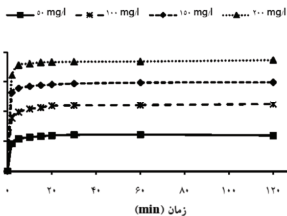
شکل ۳: اثر غلظت رنگ اسید اورانژ ۷ بر میزان جذب آن بر روی کانولا (شرایط آزمون شامل دمای ۲۰ درجه سانتی گراد، pH ۳، غلظت رنگ متغیر از ۵۰ تا ۲۰۰ میلی گرم بر لیتر، غلظت کانولا ۵ گرم بر لیتر، مدت زمان تیمار ۱۲۰ دقیق با همزدن ۱۰۰ RPM).
