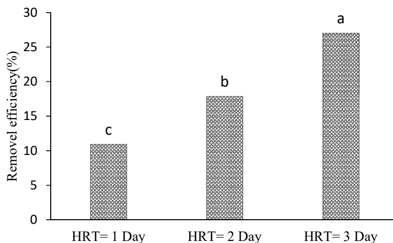
نمودار ۳- مقایسه میانگین اثر زمان ماند بر حذف نیترات (حروف متفاوت دارای اختلاف معنی‌دار)
