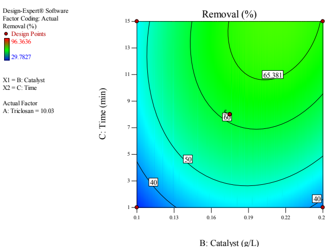
نمودار ۳- غلظت کاتالیست در برابر زمان در غلظت تری کلوسان ۱۰/۰۳ mg/L
