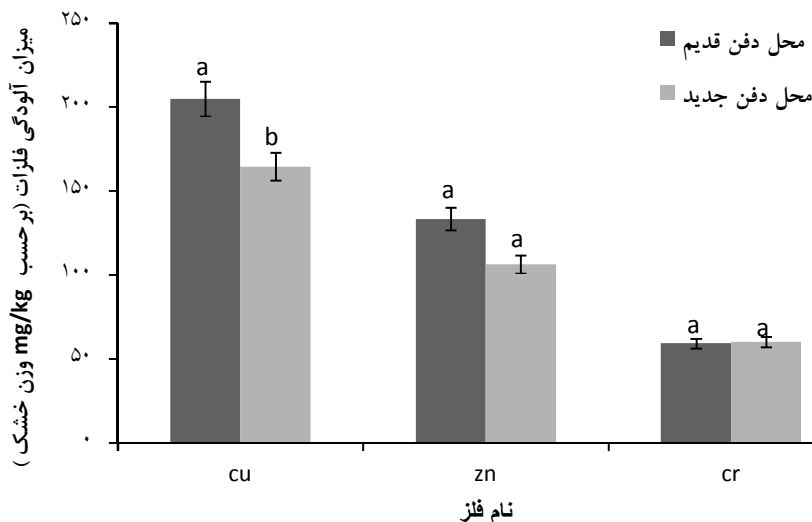
شکل ۳، میانگین مقادیر فلزات مس، روی و کروم برحسب میلی گرم بر کیلوگرم در خاک محل دفن زباله های قدیمی و جدید
