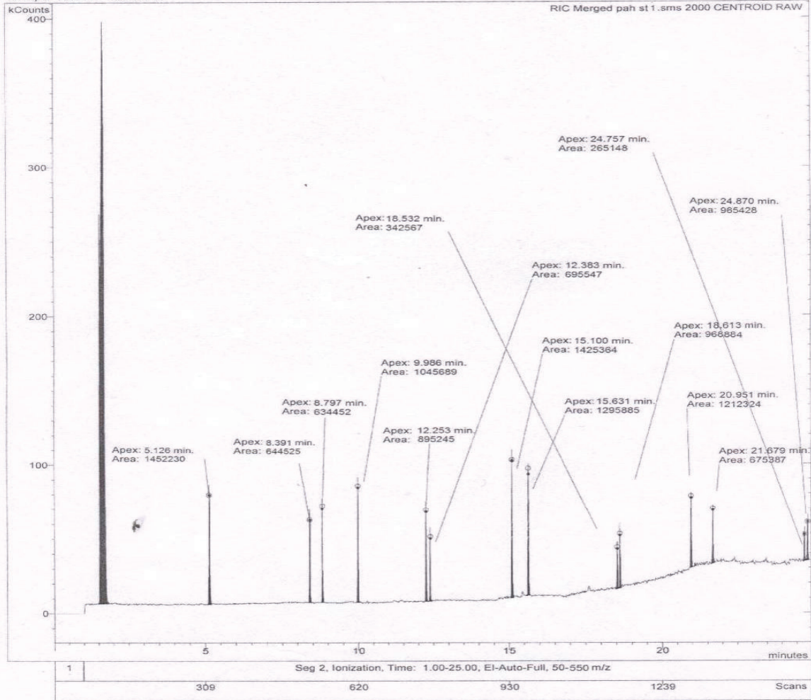
شکل ۱: کروماتوگرام محلول استاندارد
