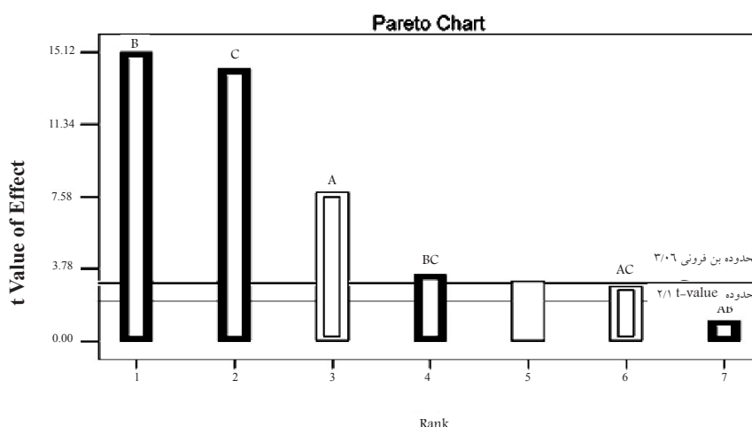
شکل ۱: نمودار pareto برای فاکتوریل کامل: (A) دانسیته تلقیح اولیه باکتریایی، (B) غلظت فنانترون در خاک و (C) نوع سورفکتانت.
