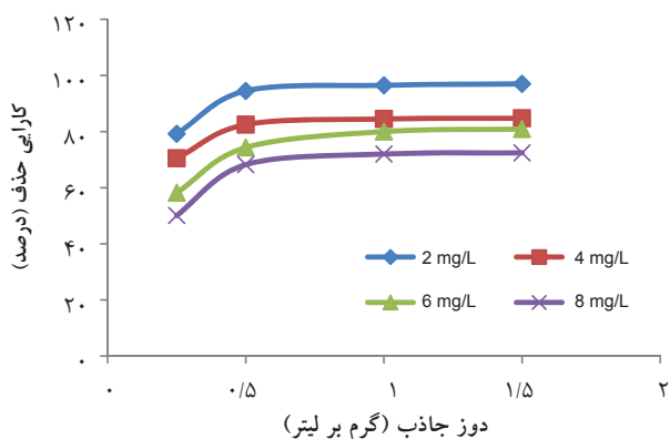
نمودار ۴- تاثیر تغییرات دوز جاذب نانوالومینا پوشش داده شده بر روی نانوتیوب کربنی چندجداره ( pH=3 زمان تماس ۴۵min )
