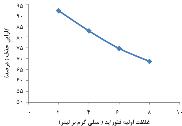
نمودار ۳- تاثیر غلظت اولیه فلوراید بر کارایی حذف توسط نانوالومینا پوشش داده شده بر روی نانوتیوب کربنی چندجداره ( pH=3 زمان تماس ۴۵min، دوز جاذب 0/5 \text{ g/L} )
