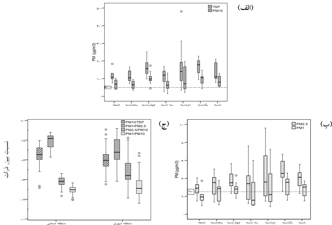
شکل ۴. تغییرات هفتگی غلظت جرمی PM_{10} و TSP (الف)، PM_{2.5} و PM_1 (ب) هوای منطقه شهری و نمودار جعبه‌ای مقادیر سالیانه نسبت‌های PM_{10}/TSP ، PM_{2.5}/PM_{10} ، PM_1/PM_{10} و PM_1/PM_{2.5} هوای منطقه شهری و صنعتی (ج)
