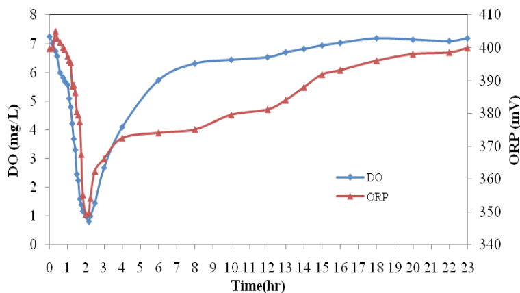
نمودار ۶- تغییرات DO و ORP در راکتور R 2 (C 0 = ۵۰ ppm)
