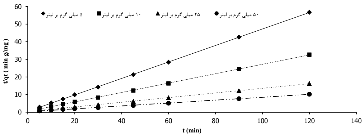
نمودار ۵: سیتیک جذب درجه دوم کاذب در حذف فنل توسط MWCNTs
