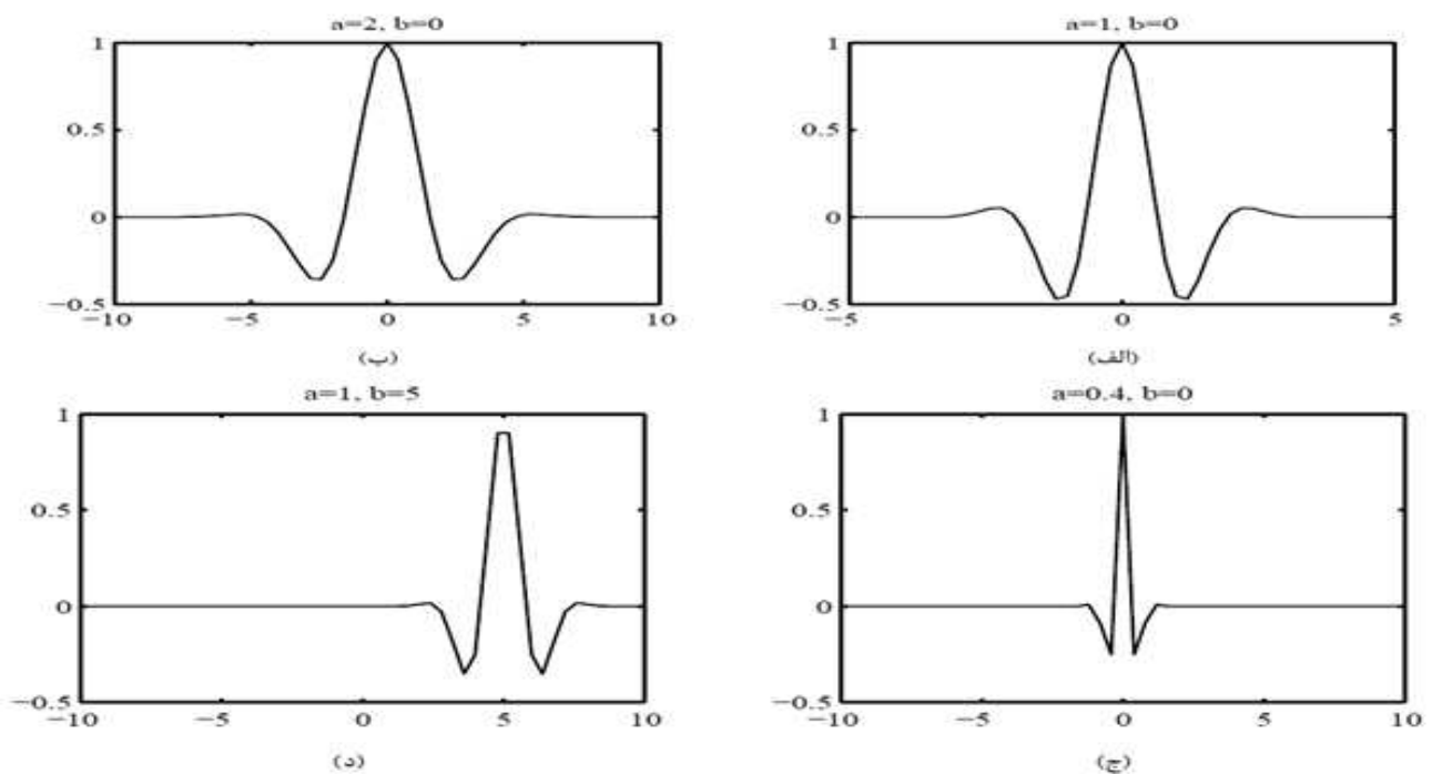
شکل ۲: موجک مورلت
