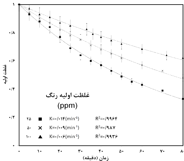
(ب) رنگ‌زدایی رنگ اسیدی سیاه ۲۶ توسط \text{TiO}_2 تثبیت شده برای مقادیر مختلف رنگ‌زا (۰/۵۲۸ mg/L \text{H}_2\text{O}_2 ، pH نرمال و غلظت آنیون: ۰ mM)
