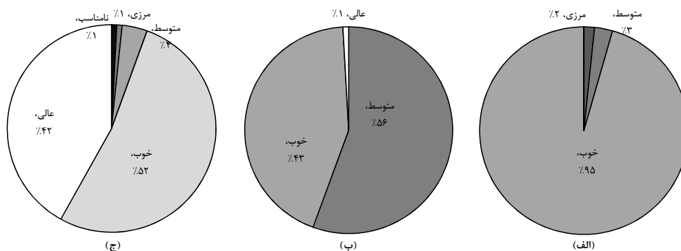
شکل ۲: طبقه بندی آب های زیرزمینی کشور (بر حسب میزان جریان) با استفاده از شاخص های (الف) MDWQI، (ب) HWQI و (ج) AWQI
