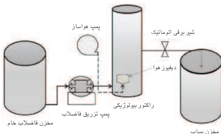
شکل ۱: شماتیک راکتور بیولوژیکی سیکیلی استفاده شده در مطالعه
