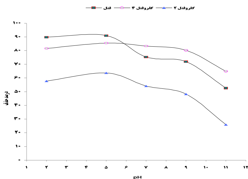
شکل ۲: تاثیر تغییرات pH بر راندمان حذف فنل، ۲-کلروفنل و ۴-کلروفنل (غلظت اولیه ترکیبات فنلی mg/L
