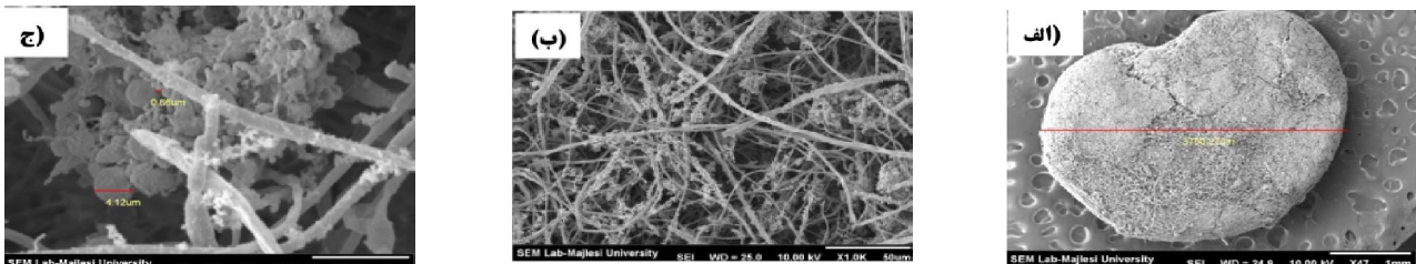
شکل ۴: گرانول بیولوژیکی با پایه تشکیل شده از باکتری‌های رشته‌ای؛ الف) گرانول کامل، ب) سطح برش خورده گرانول، ج) نمای نزدیک‌تر سطح برش خورده گرانول. (تصاویر SEM)
