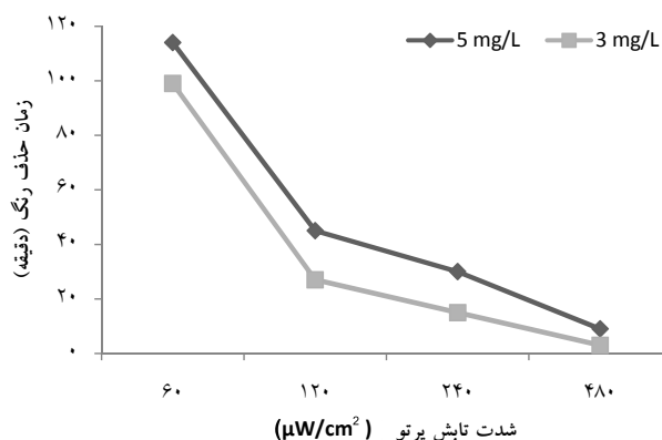
شکل ۴: حذف رنگ متیلن بلو در غلظت های ۳ و ۵ میلی گرم بر لیتر تحت تابش اشعه UVA در شدت های ۶۰ تا ۴۸۰ میکرووات بر ثانیه در حضور غلظت ۱۰۰ mg/l نانو ذرات اکسید روی
