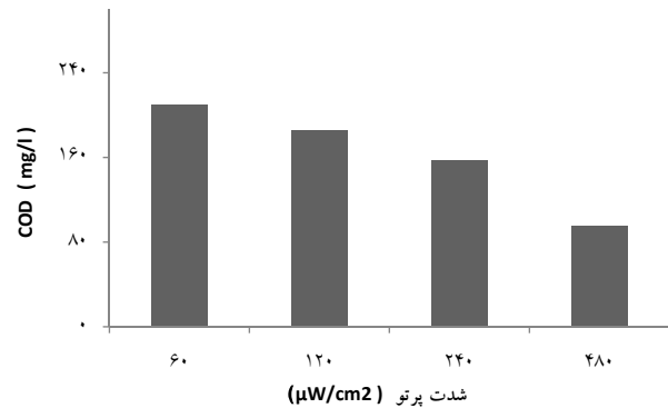
شکل ۶: کاهش COD رنگ متیلن بلو متعاقب فرایند فتوکاتالیستی با استفاده از نانو ذرات اکسید روی
