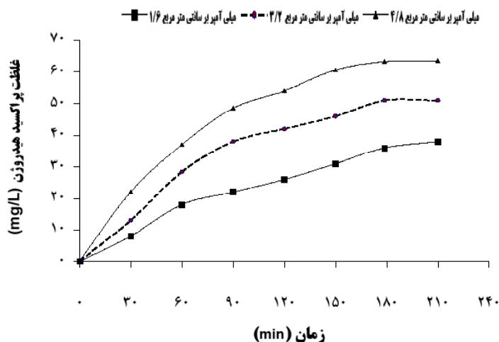
شکل ۷: مقدار پراکسید هیدروژن تولیدی در دانسیته جریان‌های مختلف (pH=۳، الکترولیت سولفات سدیم ۰.۵ mol/L، هوای ورودی ۱/۵ L/min)
